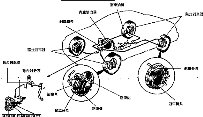
汽車剎車系統剖析圖
