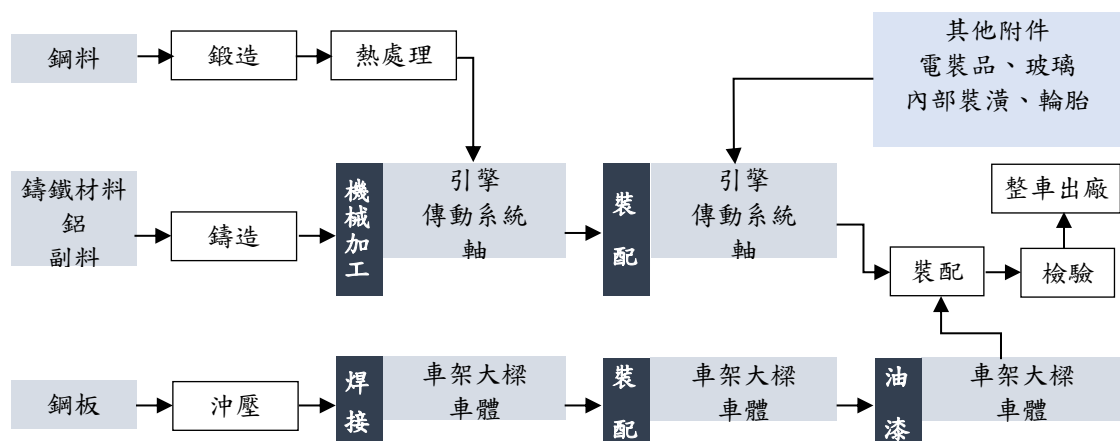
汽車及零組件製造流程
