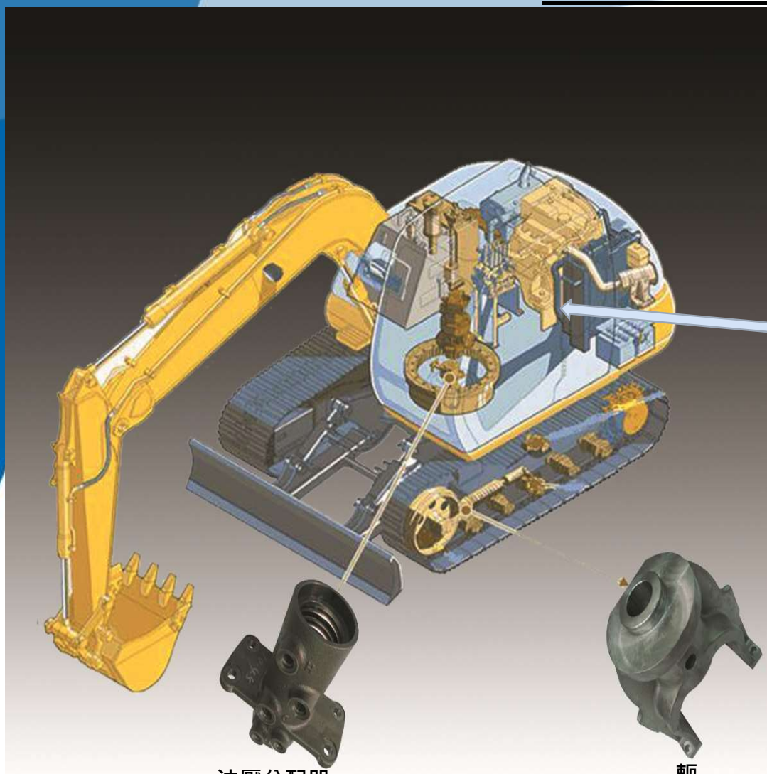
油壓分配器
