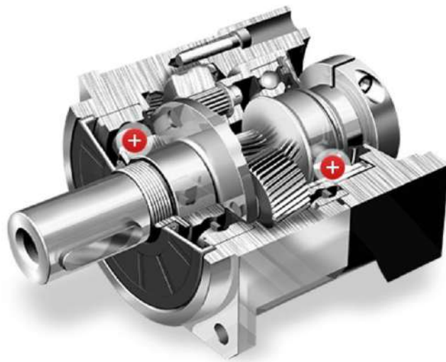
圖一：行星式減速機結構圖
