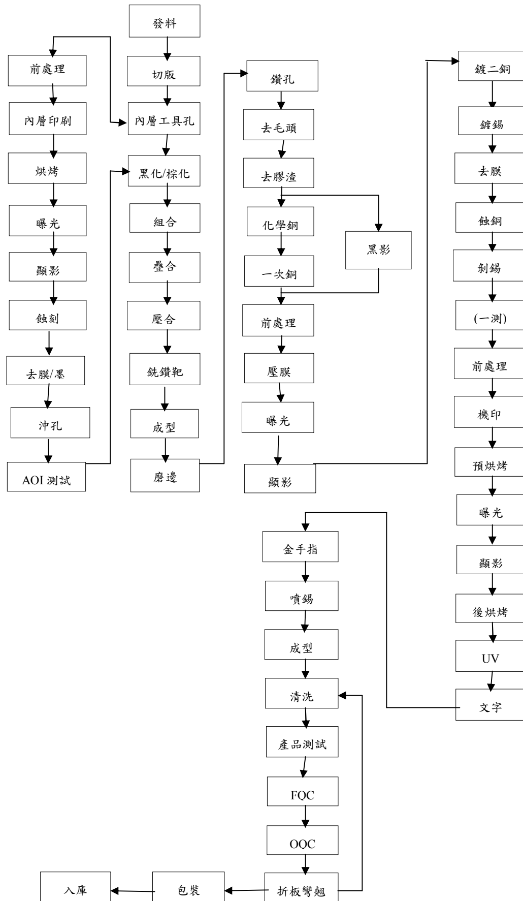
(2) 產製過程 PCB 製造流程圖
