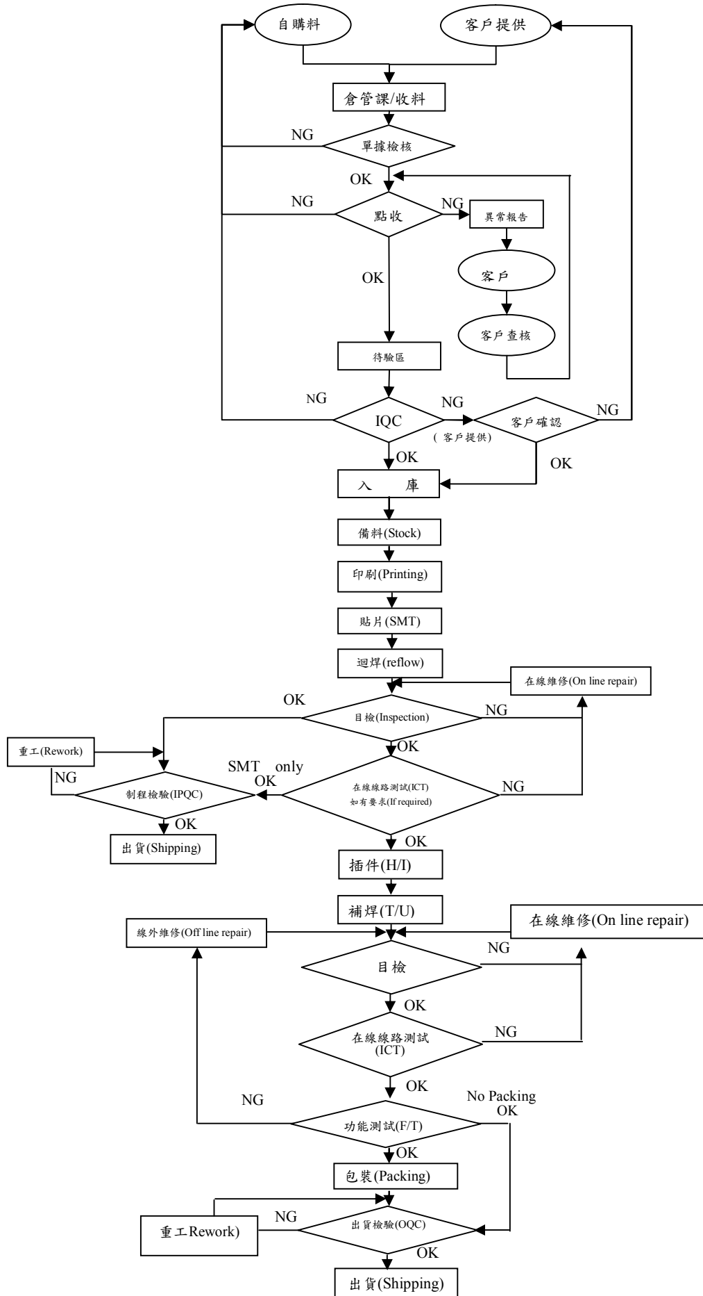
PCBA 流程圖
