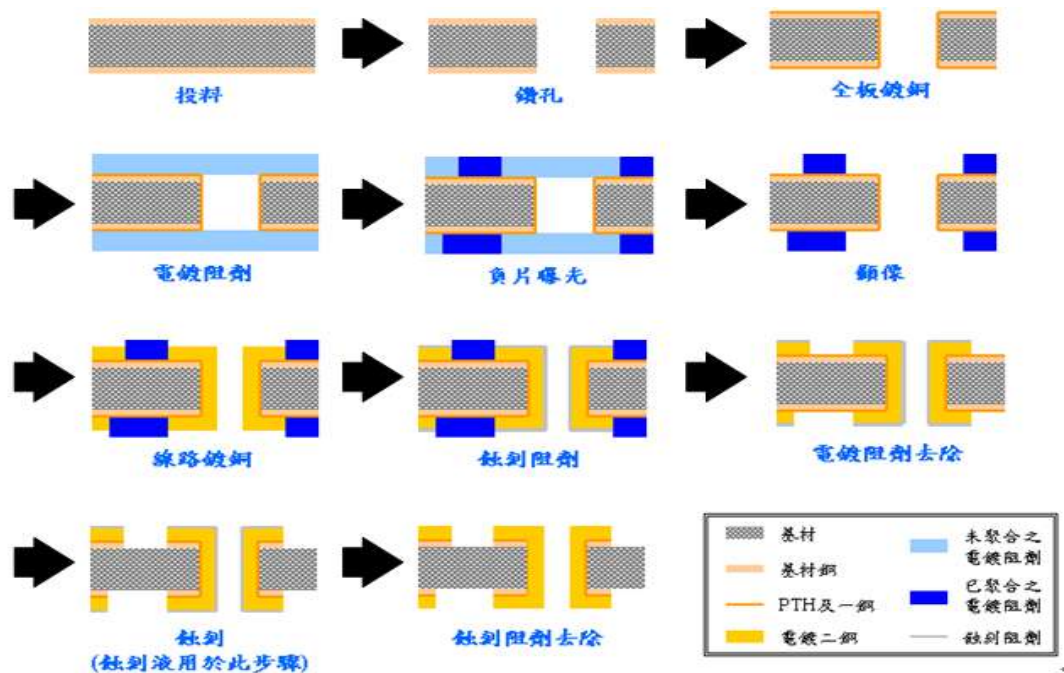
圖 1.常見的電路板線路製作流程(Pattern process)
