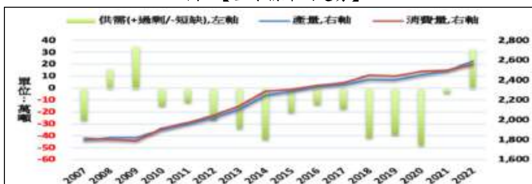
圖 6【全球精煉銅趨勢】
