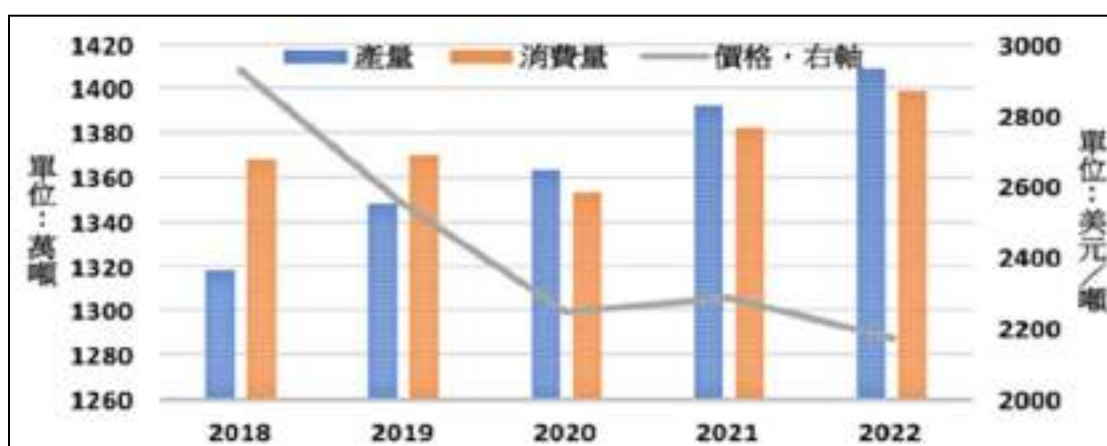
圖 7【全球精煉鋅供需及價格趨勢】
