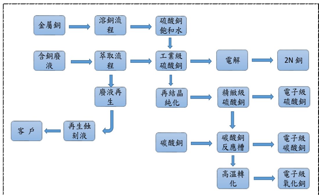
圖 2. 再生銅鹽產品產製流程
