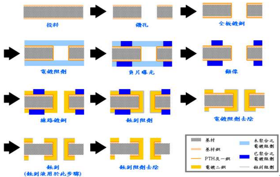
圖 1.常見的電路板線路製作流程(Patternprocess)
