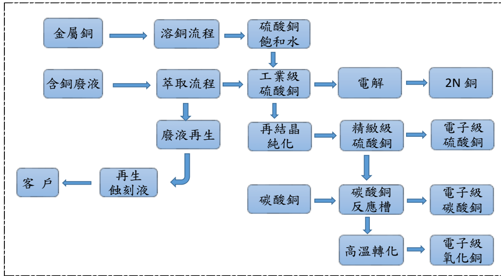
圖 3.再生銅鹽產品產製流程
