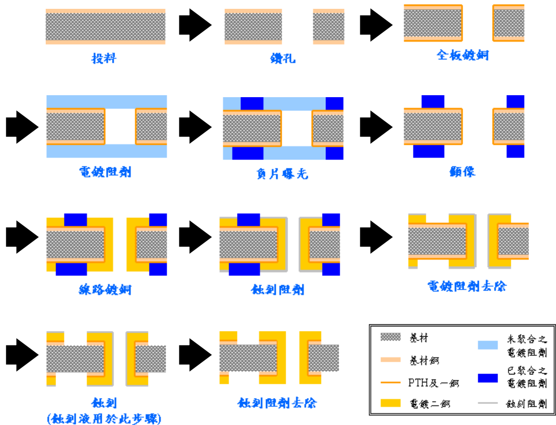
圖 1.常見的電路板線路製作流程 (Patternprocess)
