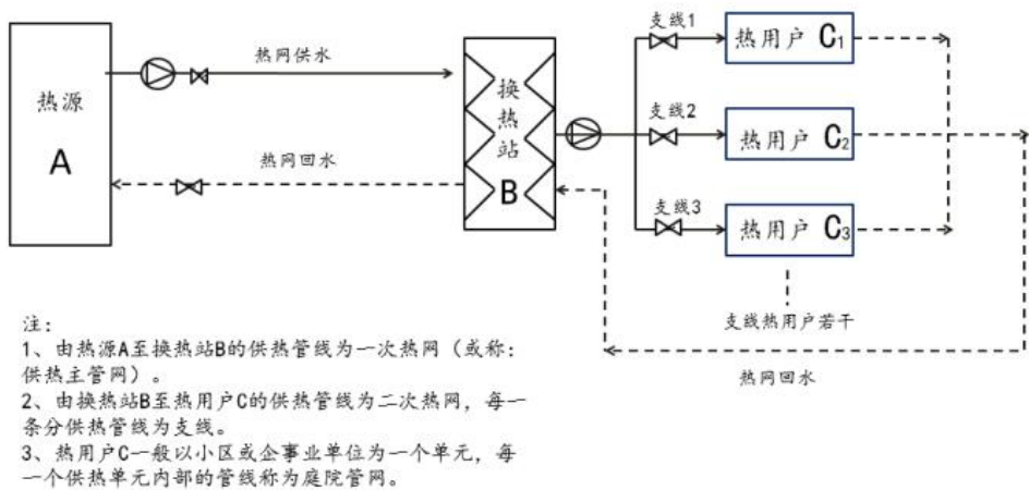
热电联产供热流程图
