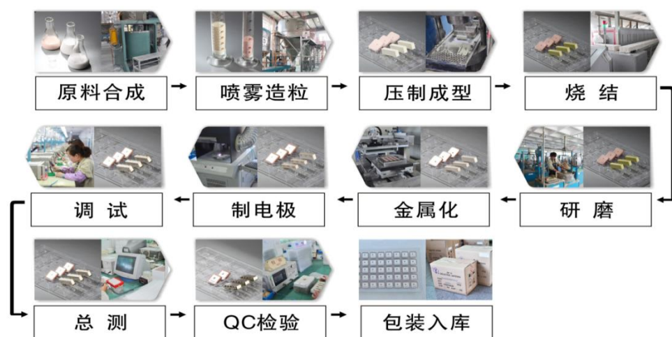
⑤EOC双工器生产工艺流程
