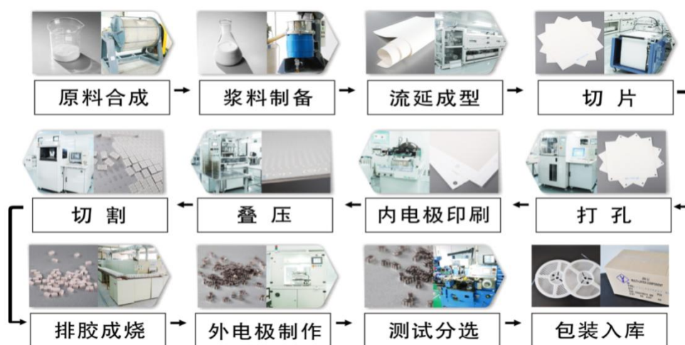
④高温烧结陶瓷元器件生产工艺流程
