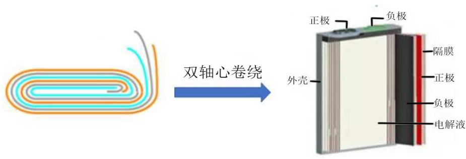
图 方壳电池结构
