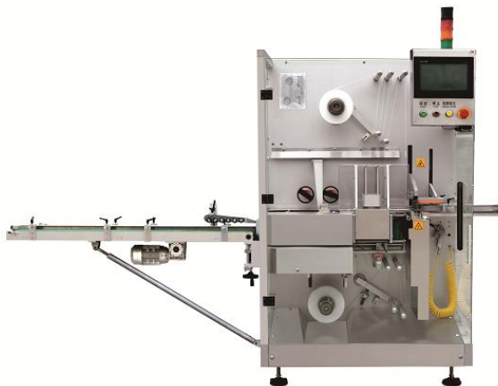
图 3：BC240 缠绕式薄膜包装机
