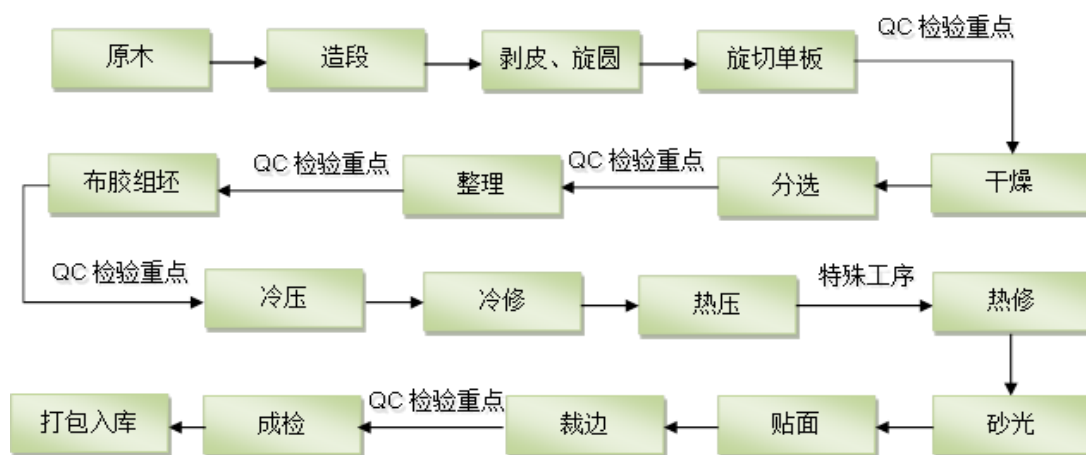
装饰板及建筑模板工艺流程图
