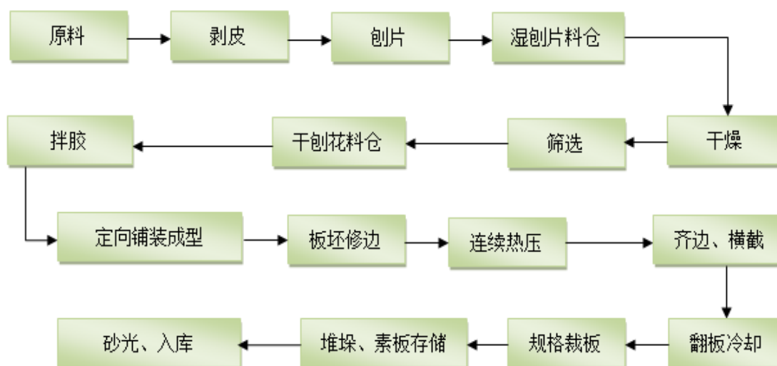
COSB 工艺流程图
