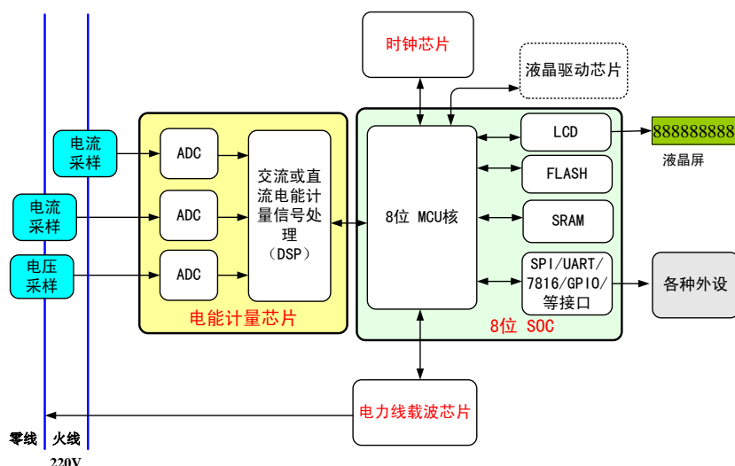
当前国网智能电表分立器件方案系统示意图
