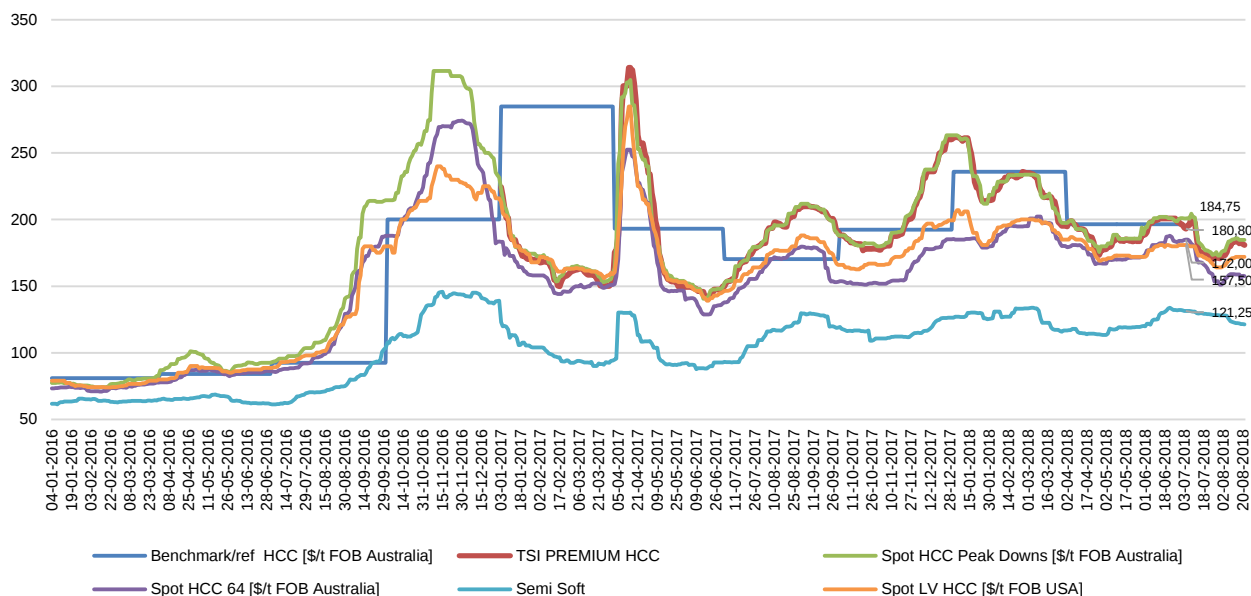
Wykres 3. Benchmarkowe i spotowe notowania cen węgla koksowych ($/t FOB)
