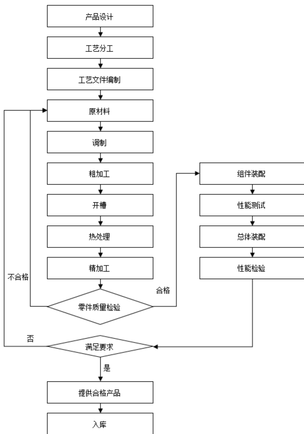
(3) 非航空液压系统工艺流程图
