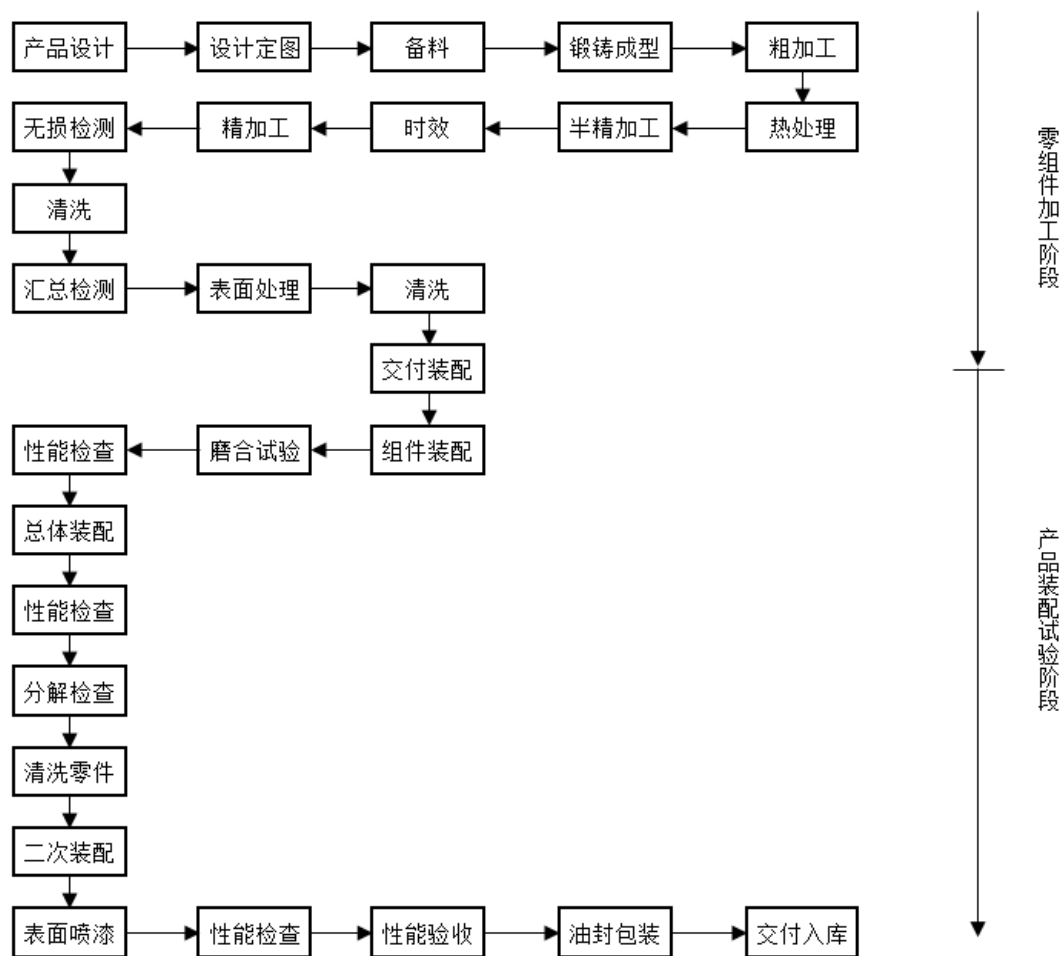
(2) 非航空产品工艺流程图
