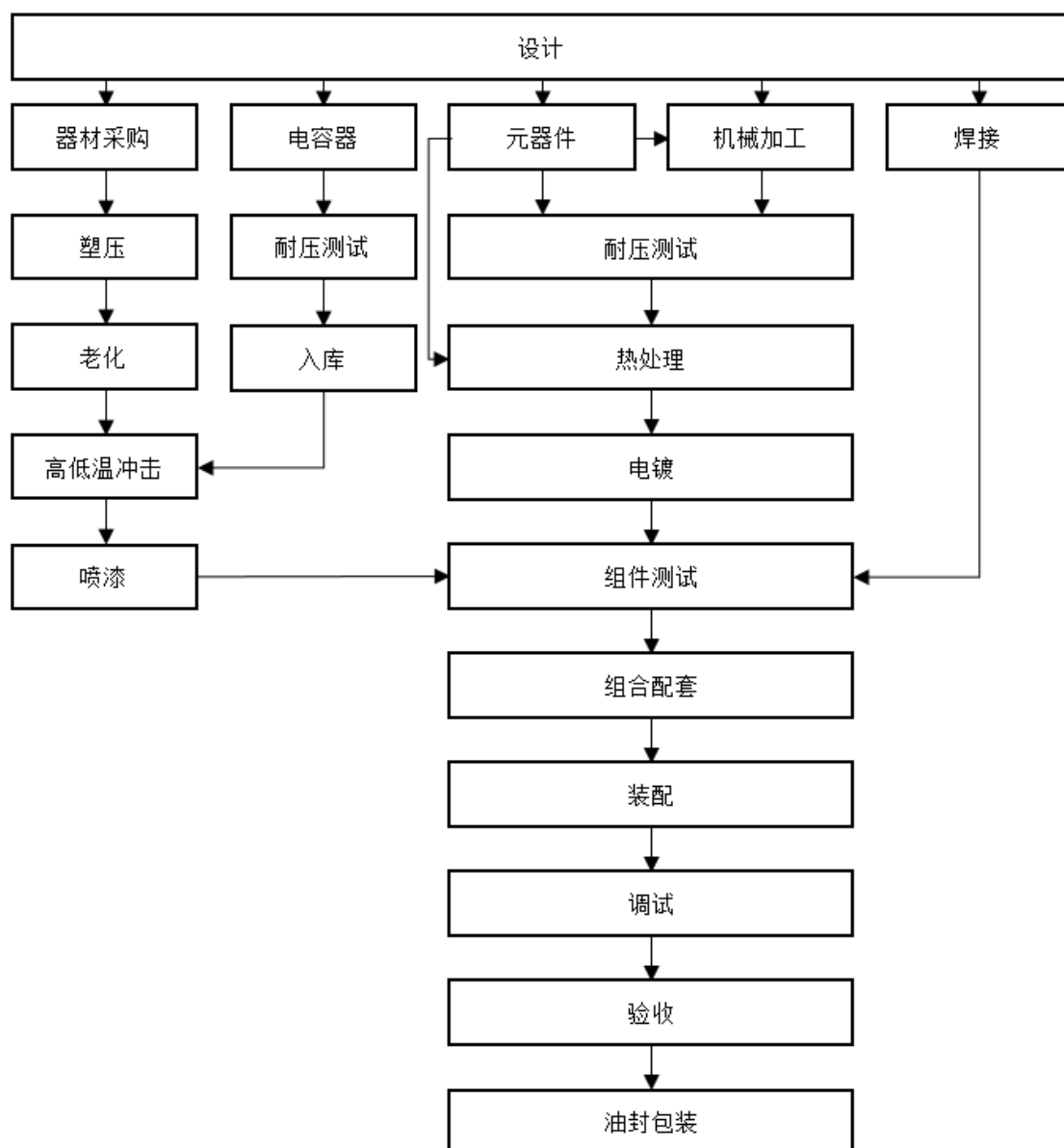
(3) 航空地面检测试验设备工艺流程图
