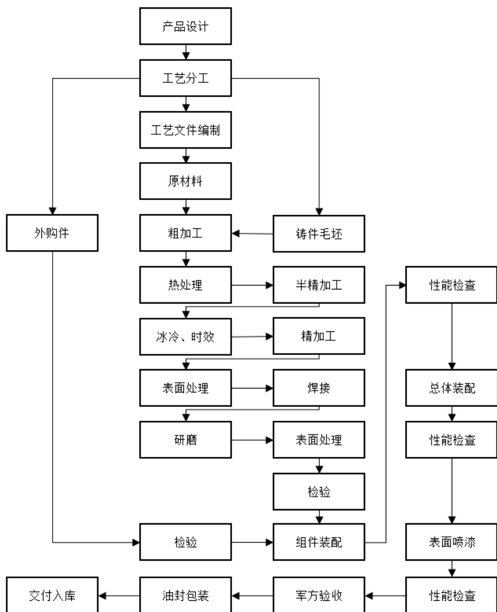
(2) 非航空液压元件工艺流程图
