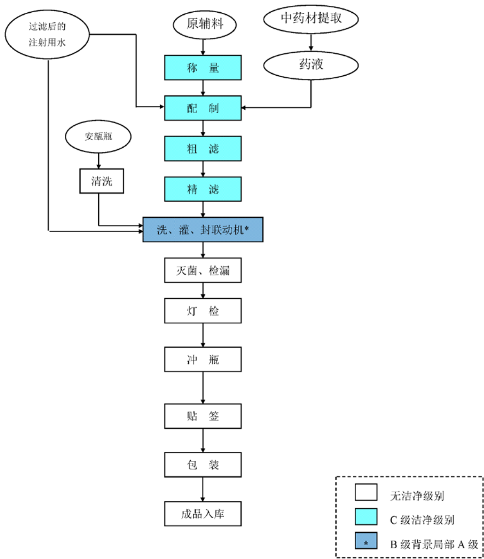
(4) 针剂工艺流程图
