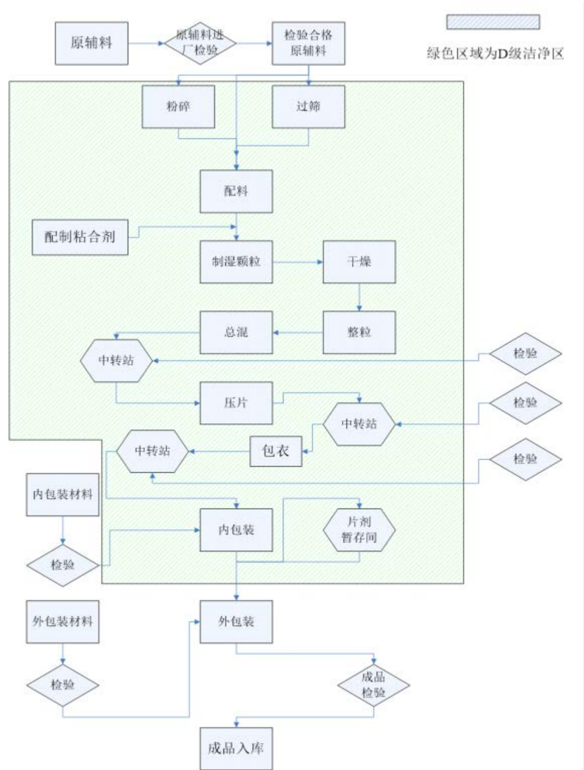
(2) 包衣片工艺流程图
