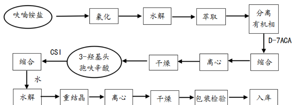
(6) 头孢呋辛酸生产流程图
