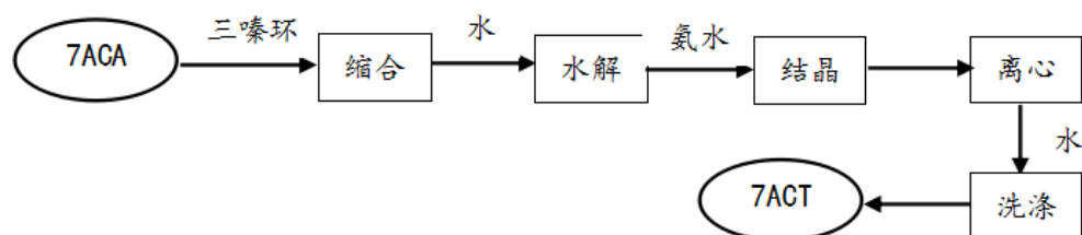
2) 头孢曲松钠（非无菌粉）生产流程图
