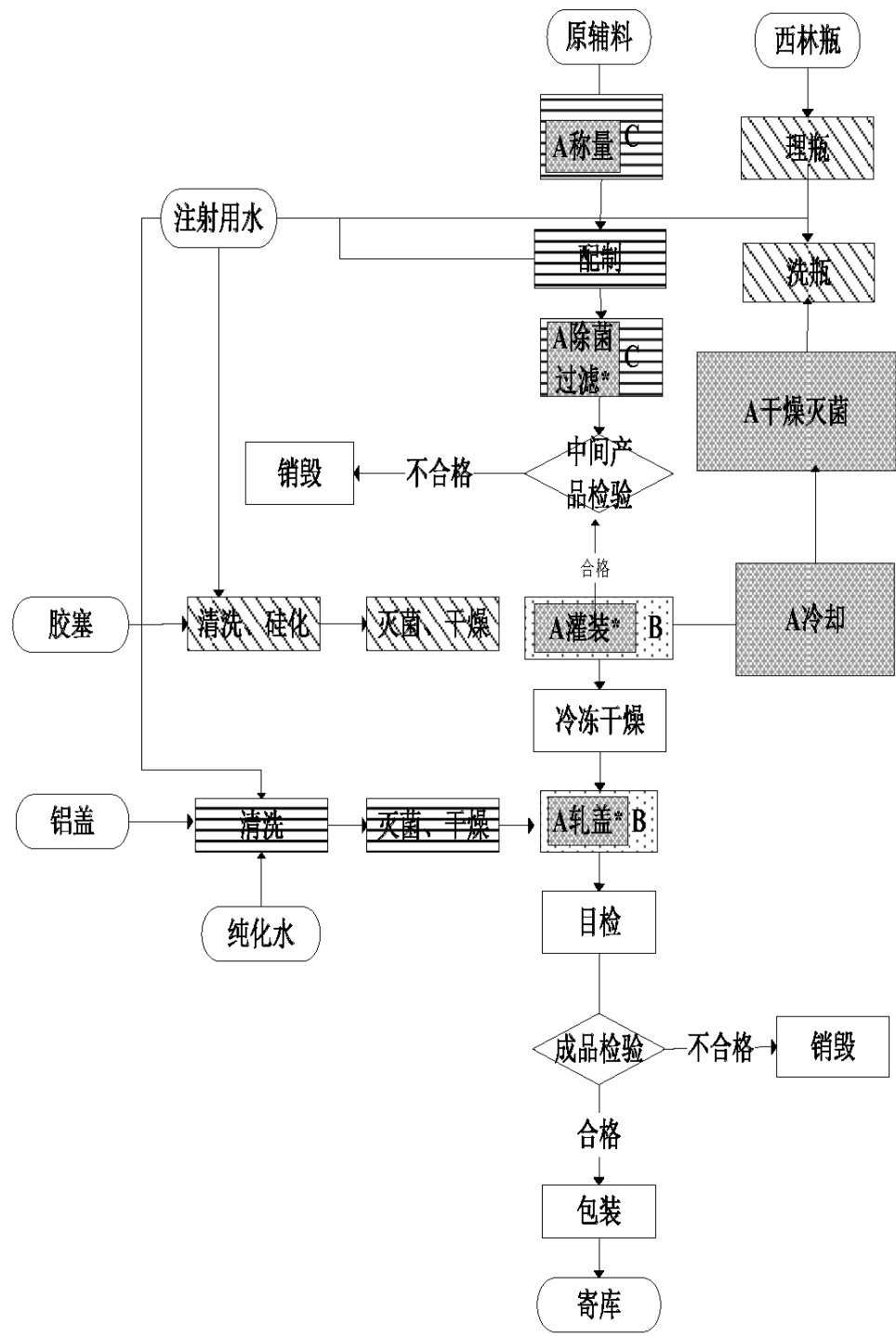
(4) 普药冻干粉针工艺流程图
