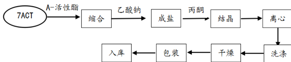
(5) 阿莫西林生产流程图
