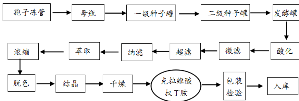
(3) 克拉维酸钾生产流程图
