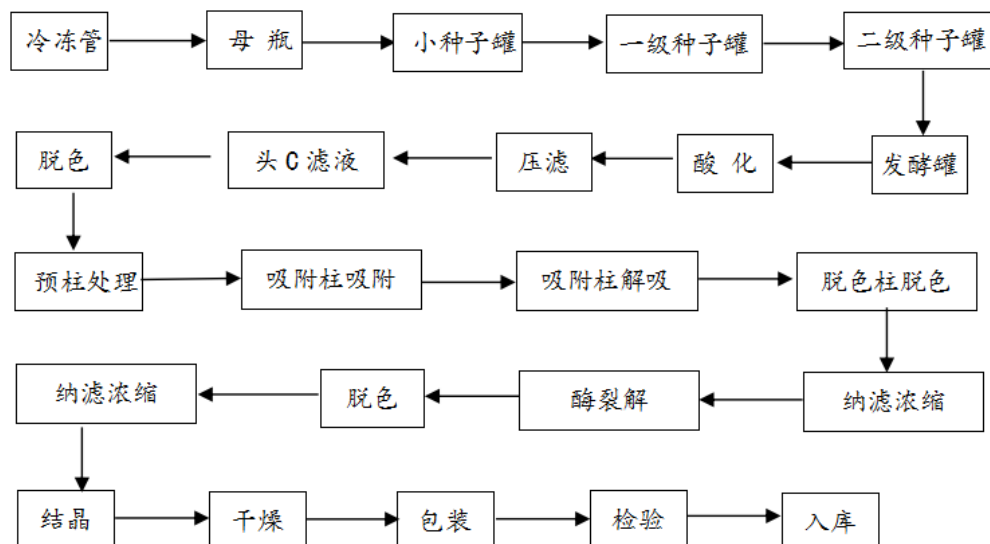
(2) 克拉维酸叔丁胺生产流程图
