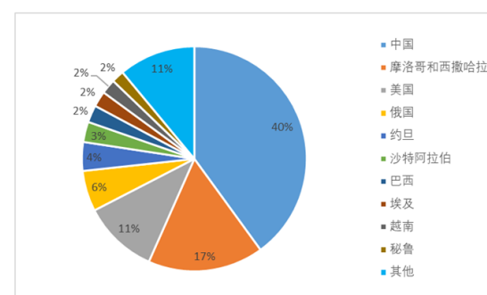
全球磷矿石产量分布
