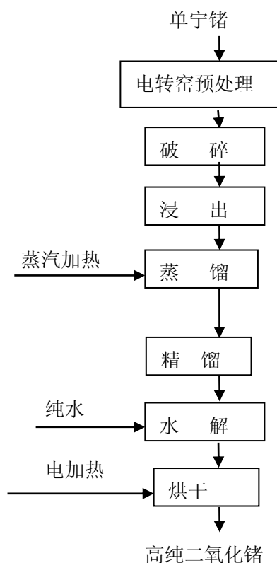
高锗流程图
