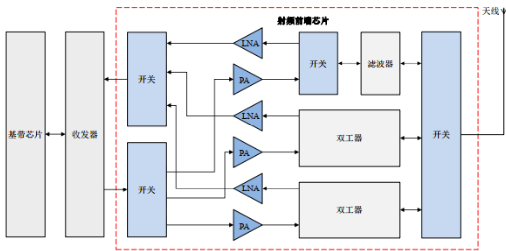
智能手机通信系统结构示意图
