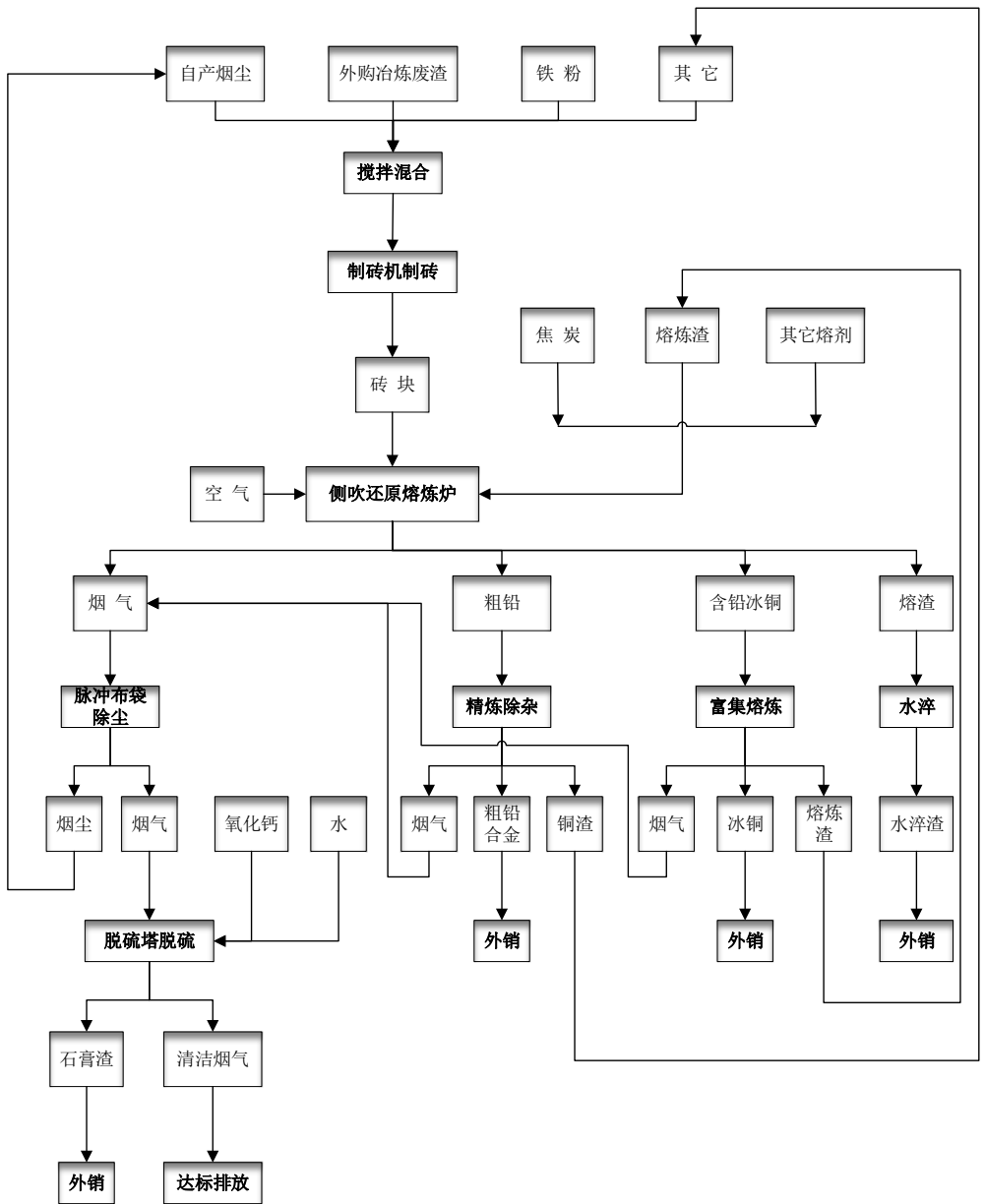
靖远宏达工艺流程图如下：
