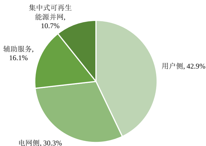
中国新增投运电化学储能项目应用分布
