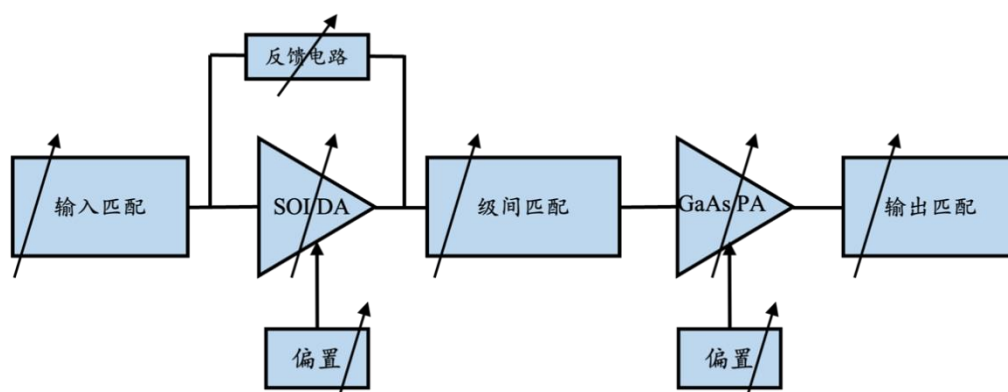
公司可重构技术路线的4G MMB功率放大器芯片原理示意图（以其中一路通路为例）
