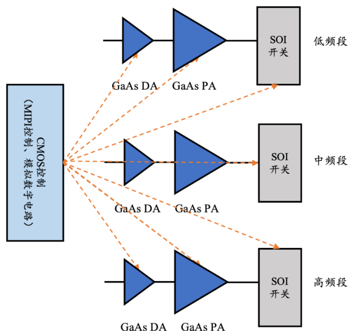
传统技术路线的4G MMB功率放大器模组原理示意图
