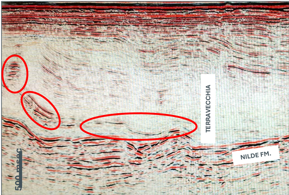
TERRAVECCHIA OUTCROP EXAMPLES
