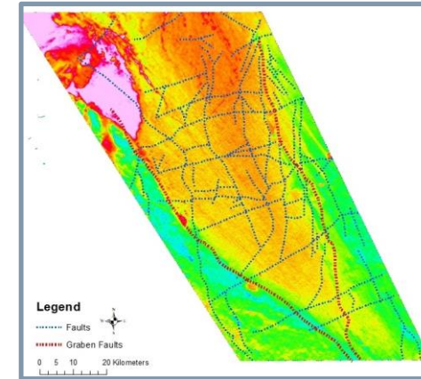
Radiometric Interpretation (K)
