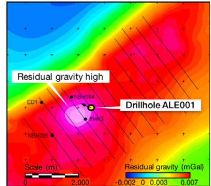
Gravity survey
