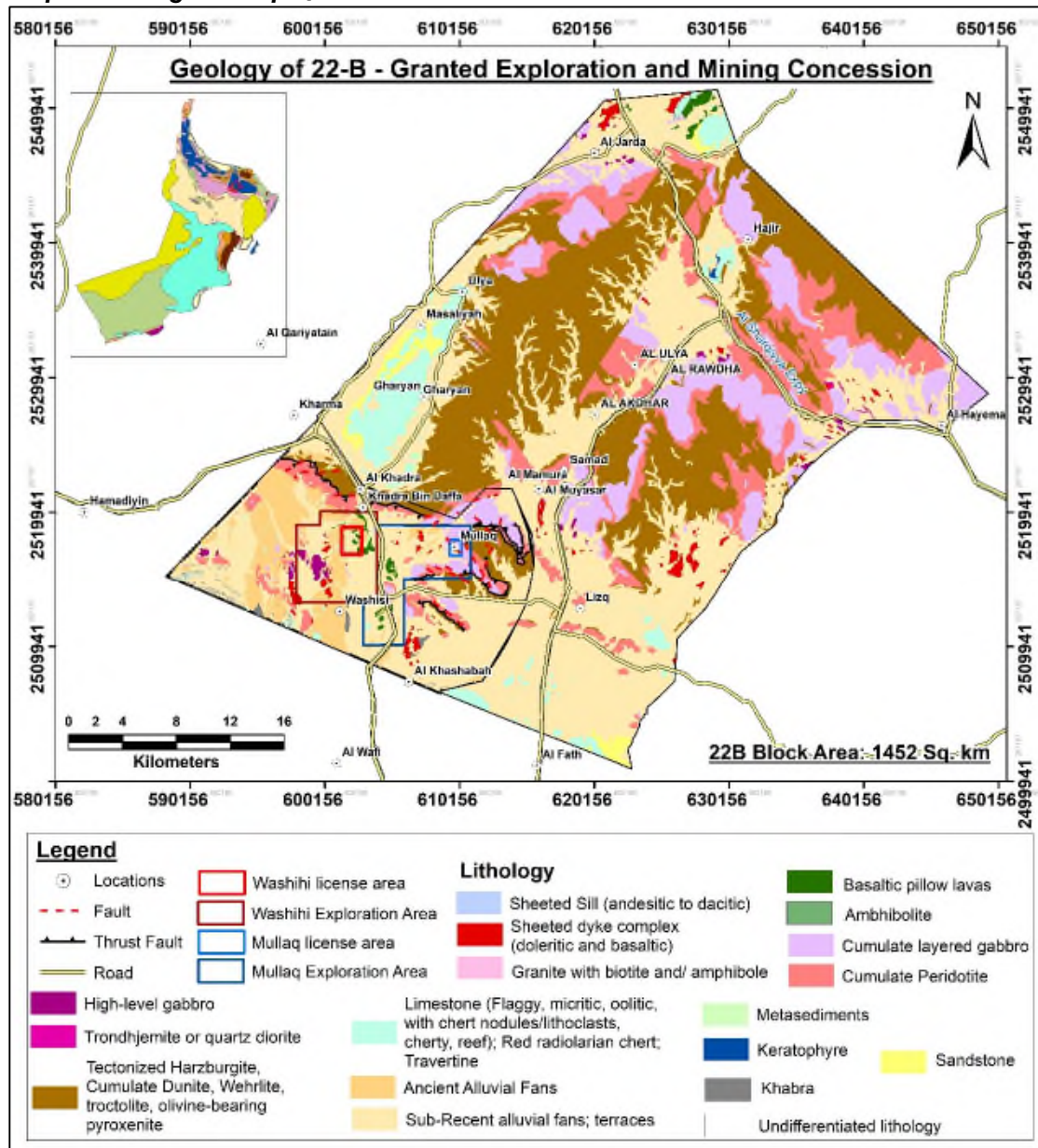
Map2 – Geological Map of Block 22-B
