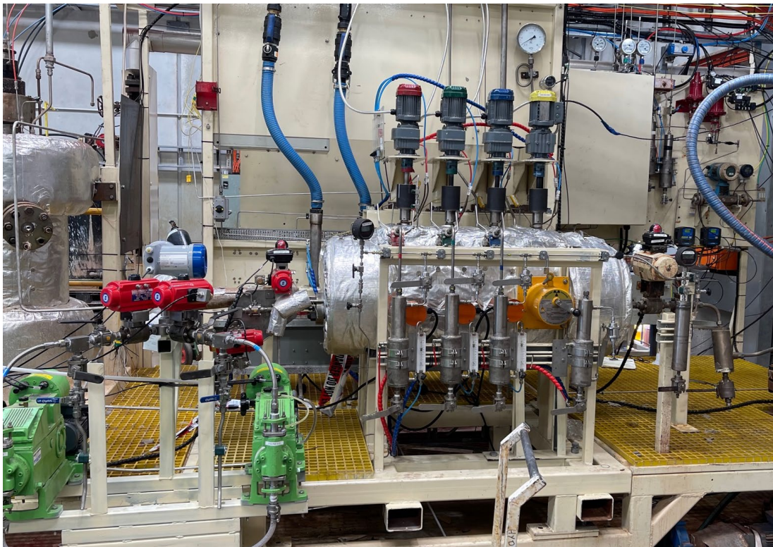
Figure 3: Pressure Leaching in Autoclave at ALS
