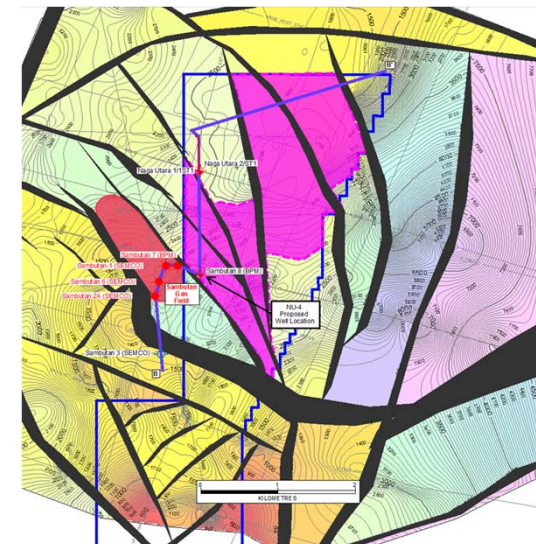
Naga Utara Depth Map - Top Pro Delta
