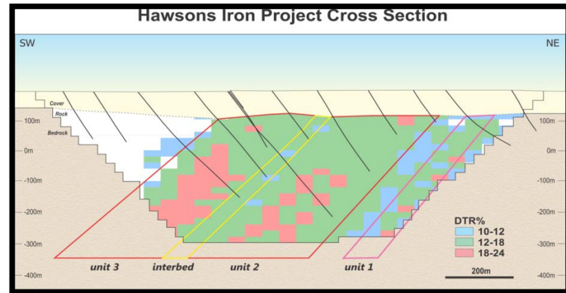
magnetite
