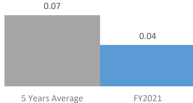
EPS ($ CENTS)
