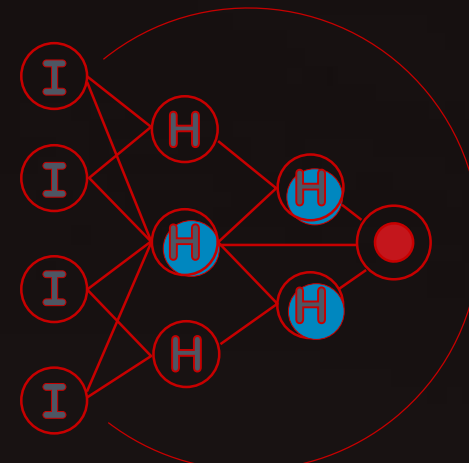
למידת מכונה
