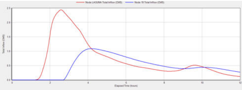
Figura 2: Caudal de entrada y salida espacio de laminación I, para la lluvia de 72mm
