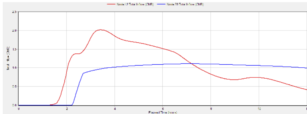
Figura 3: Caudal de entrada y salida espacio de laminación II, para la lluvia de 72mm
