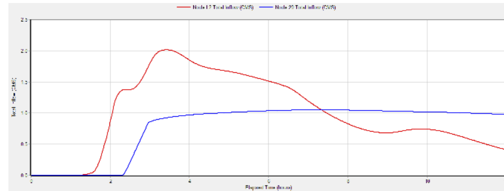
Figura 4: Caudal de entrada y salida espacio de laminación II, para la lluvia de 83mm
