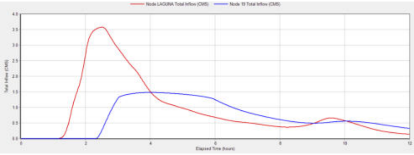
Figura 3: Caudal de entrada y salida espacio de laminación I, para la lluvia de 83mm
