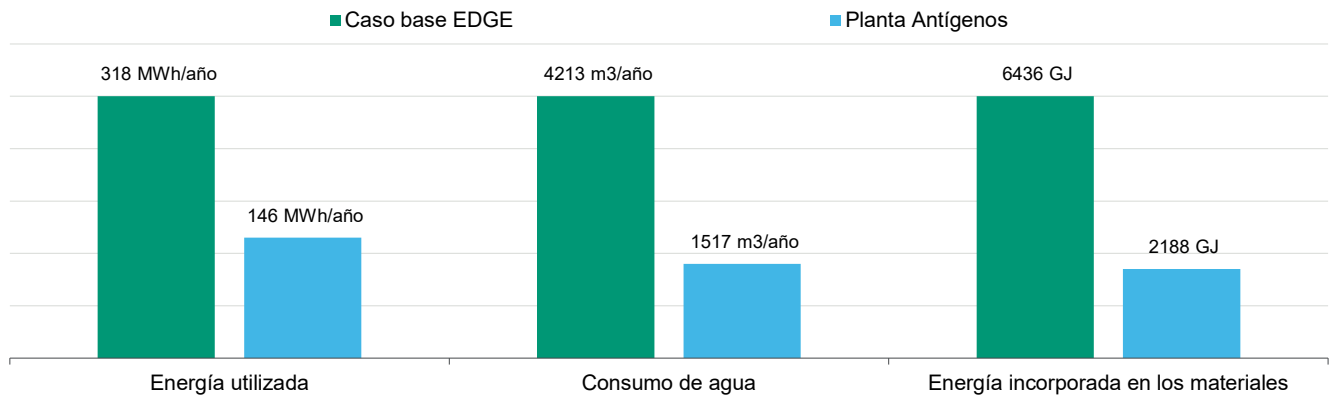
Figura 1: Utilización de energía, agua y energía incorporada en los materiales de la Planta Mercedes Tecnovax
