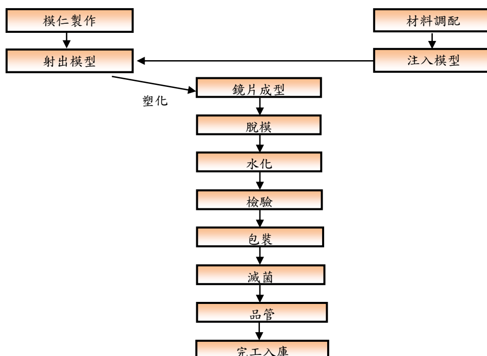
拋棄式軟式隱形眼鏡注模式加工流程
