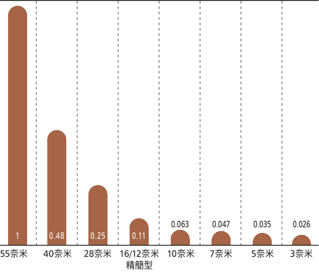
不同技術的產品晶粒大小比較
