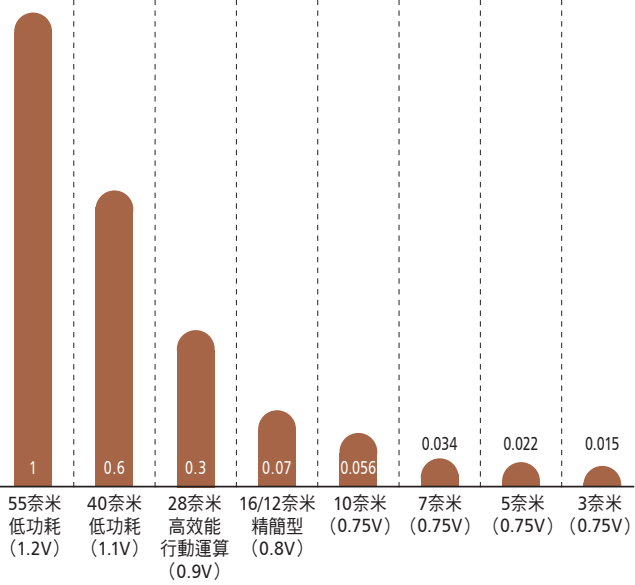
不同技術的產品使用耗電比較
