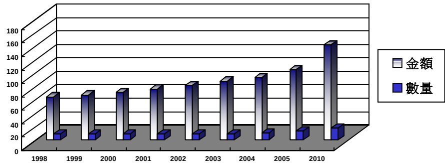
圖二 1998~2010年車用感測器市場銷量與金額統計
