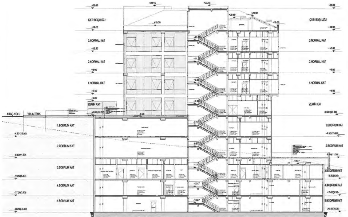
2-2 KESİTİ ÖLÇEK :1/100
