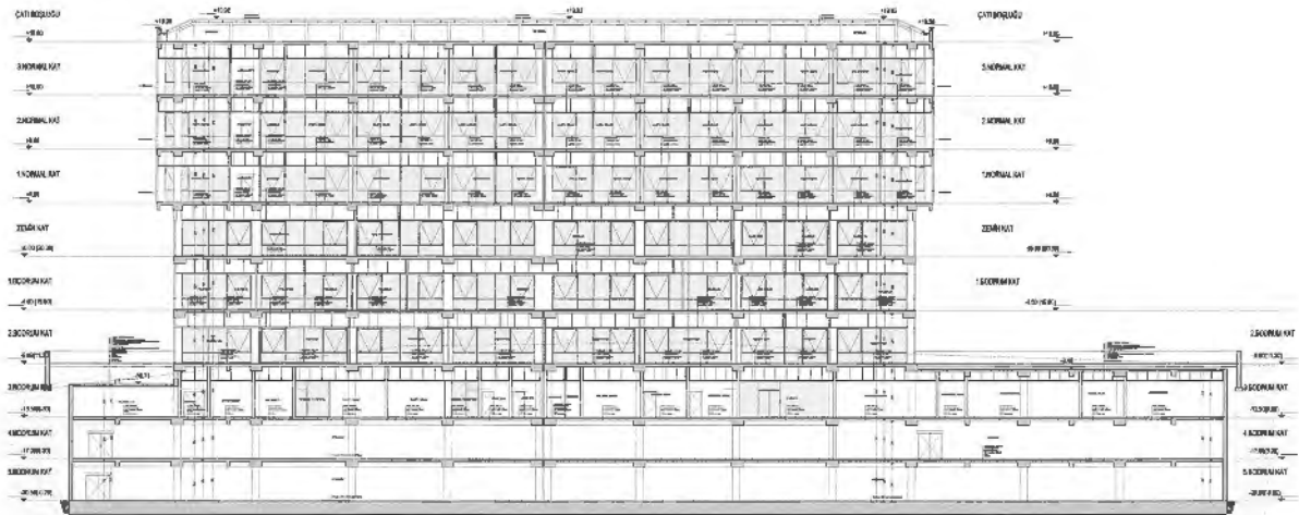
4-4 KESİTİ ÖLÇEK :1/100
