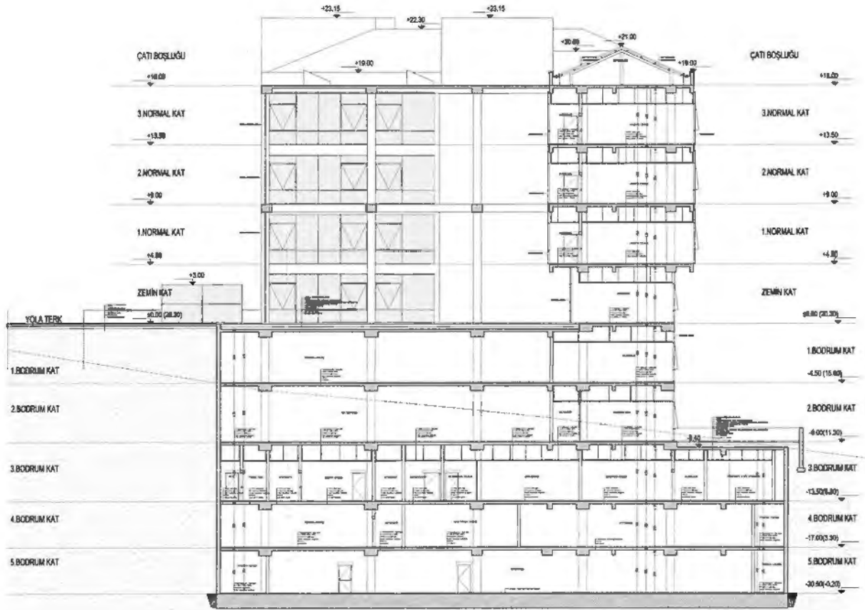
3-3 KESİTİ ÖLÇEK :1/100
