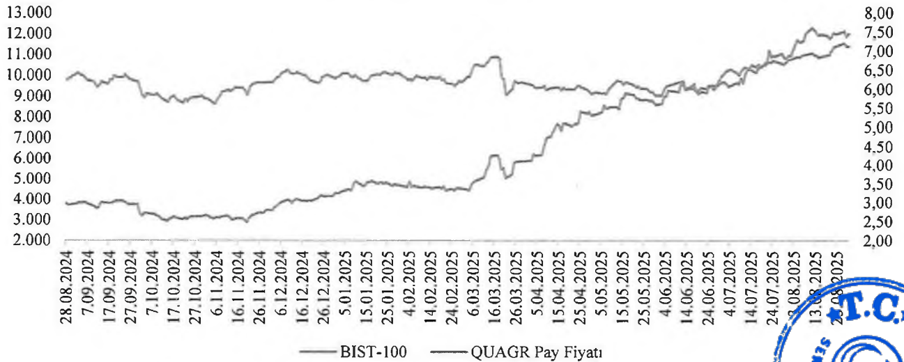
QUAGR/BIST100 Grafik
