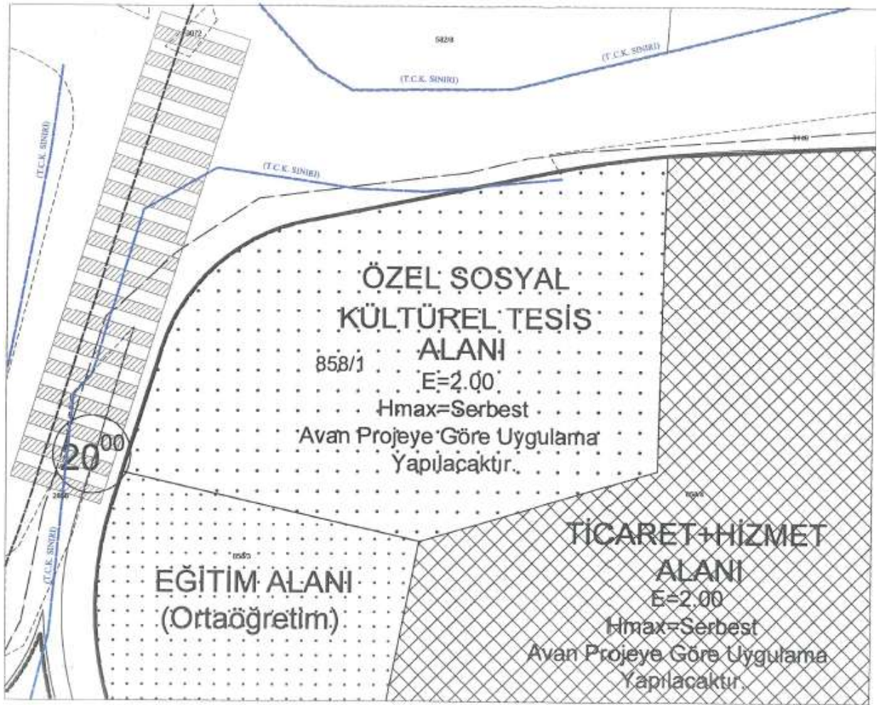
İmar Plan Örneği
