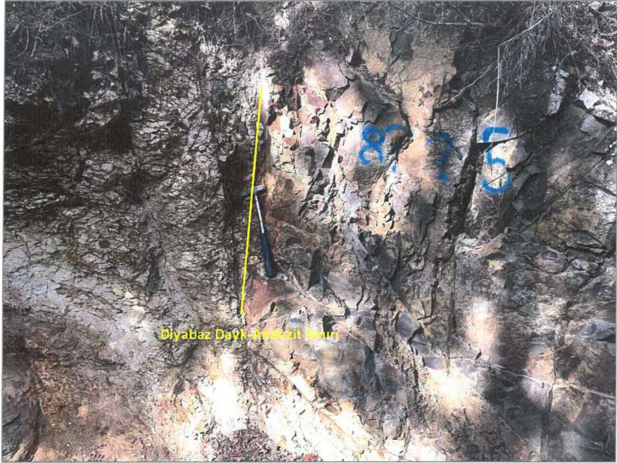
Şekil- 27. Sarıalan Altın, Gümüş Proje Alanı İçerisindeki Diyabaz Dayk-Andezit Konağı
