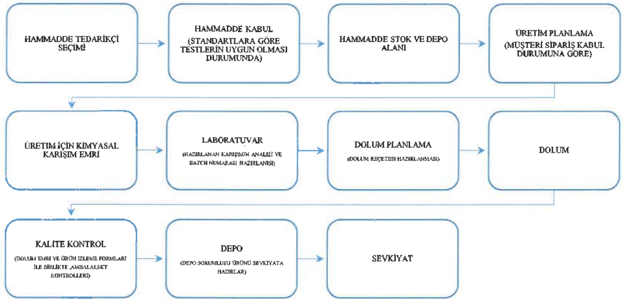
Şekil: Üretim Akış Şeması
