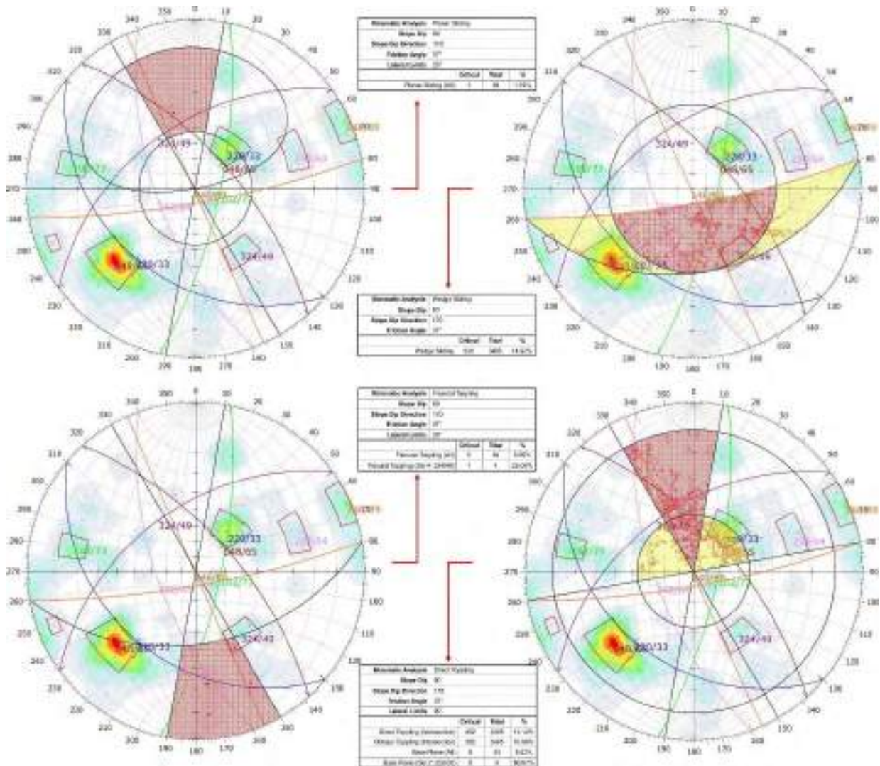
Şekil 106 Kinematik analizlerden bir örnek (170/80 yönelimli şev için)
