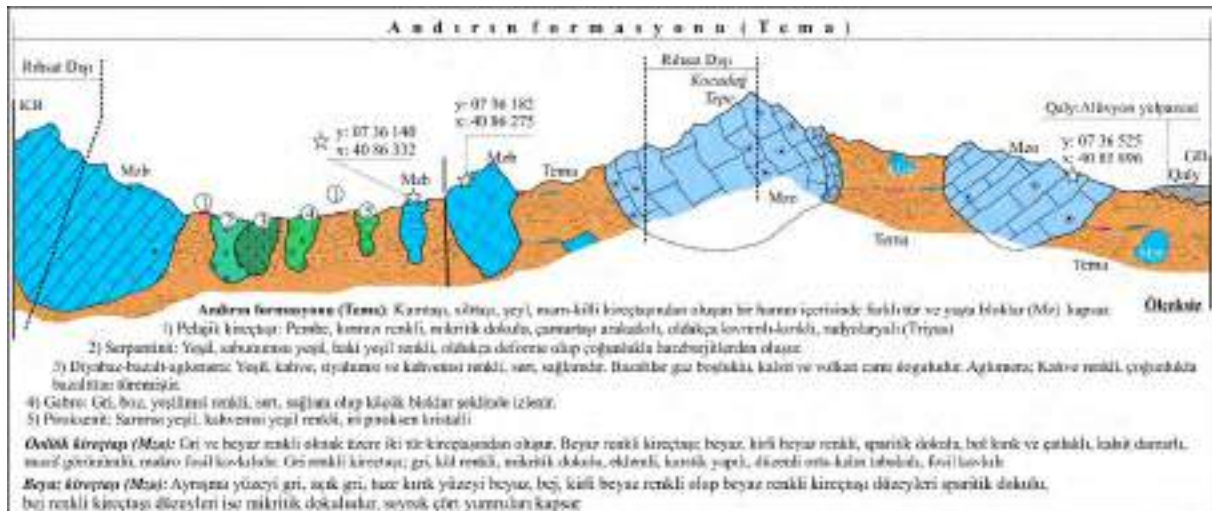
Şekil 49 Andırın Formasyonu ile birimin içerisindeki blokların ilişkisini gösteren stratigrafik enine kesit.
