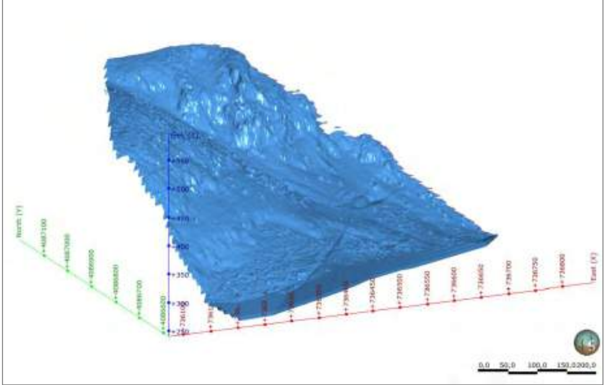
Şekil 13 Kuzey toplam hacim görseli.
