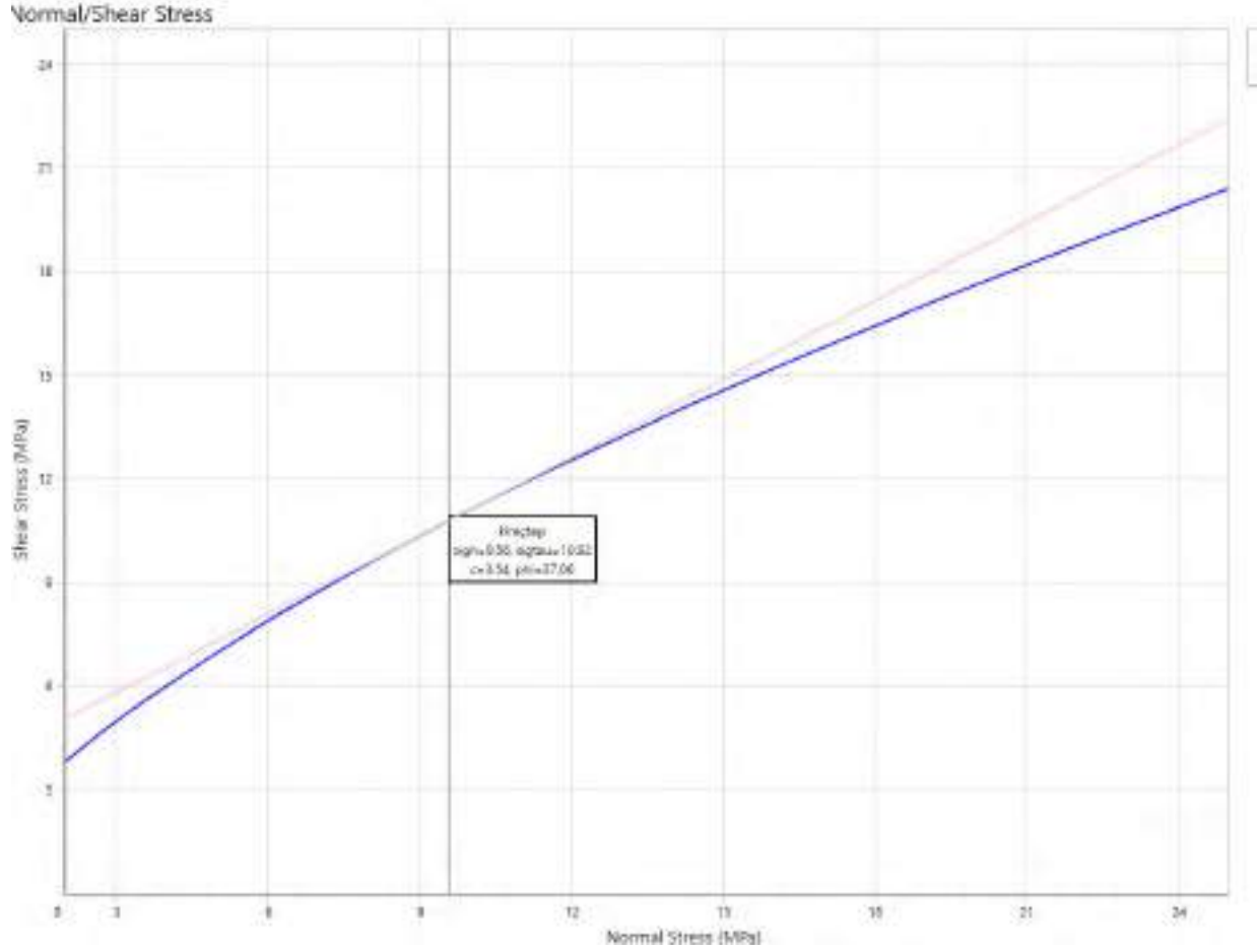
Şekil 101 Hoek- Brown yenilme ölçütüne göre hazırlanan kütsel yenilme zarfı.
