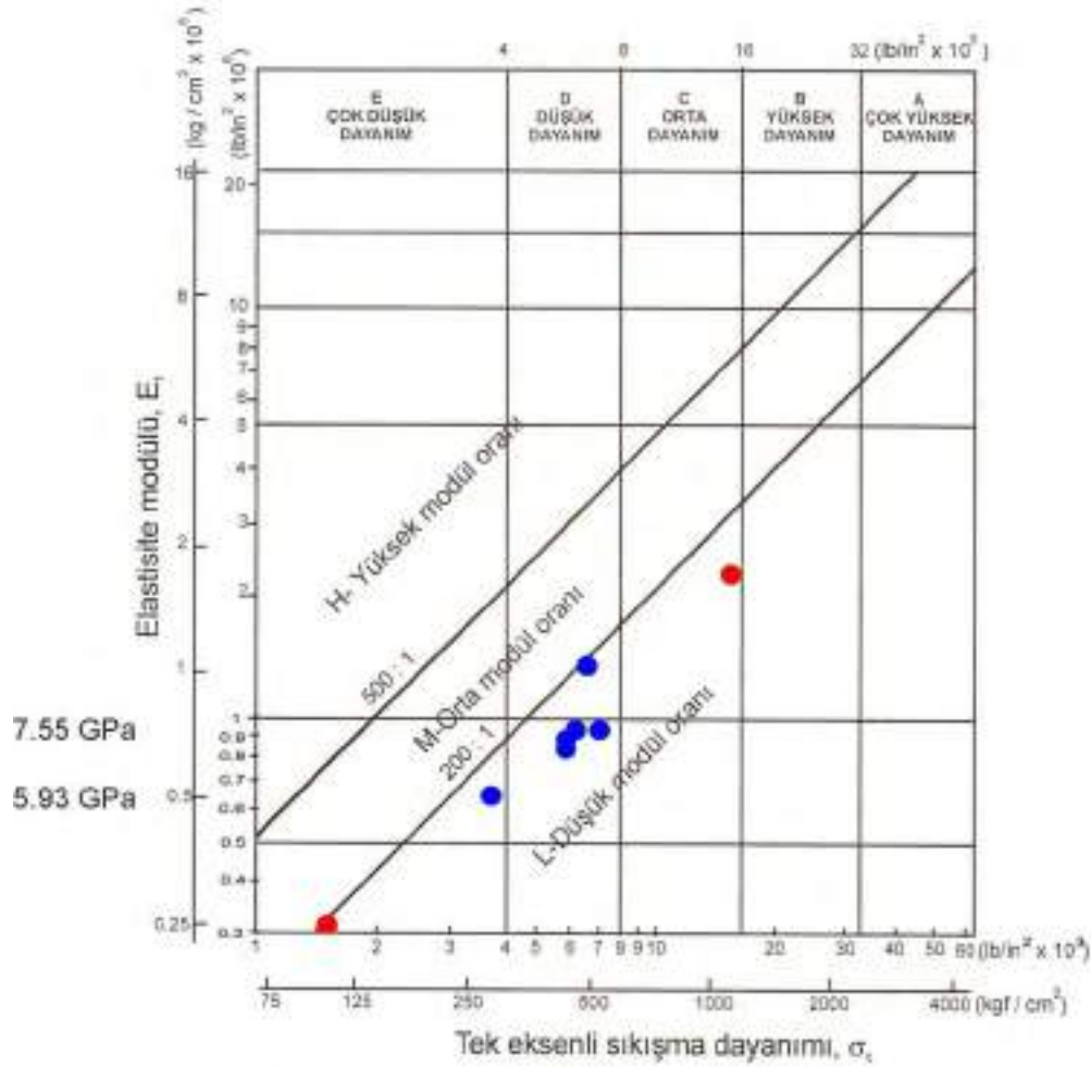
Şekil 92 Farklı kaya sınıflamalar göre kireçtaşlarının konumu.
