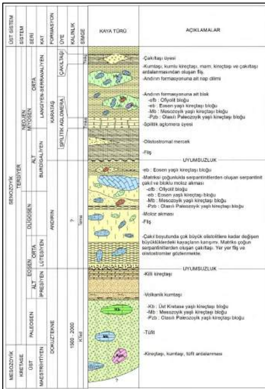
Şekil 44 Misis istifinin genelleştirilmiş stratigrafi kesiti (Bilgin, 2013).
