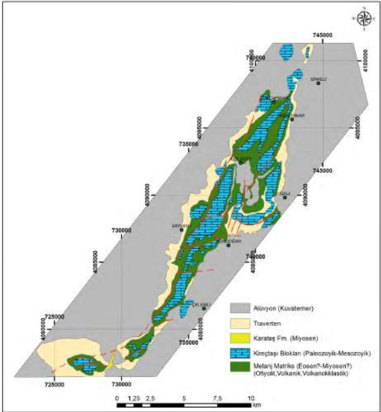
Şekil 55 Çalışma alanı ve yakın çevresinin tektonik haritası (Ünlüoğlu ve Akıncı, 2017' den değiştirilerek alınmıştır.).
