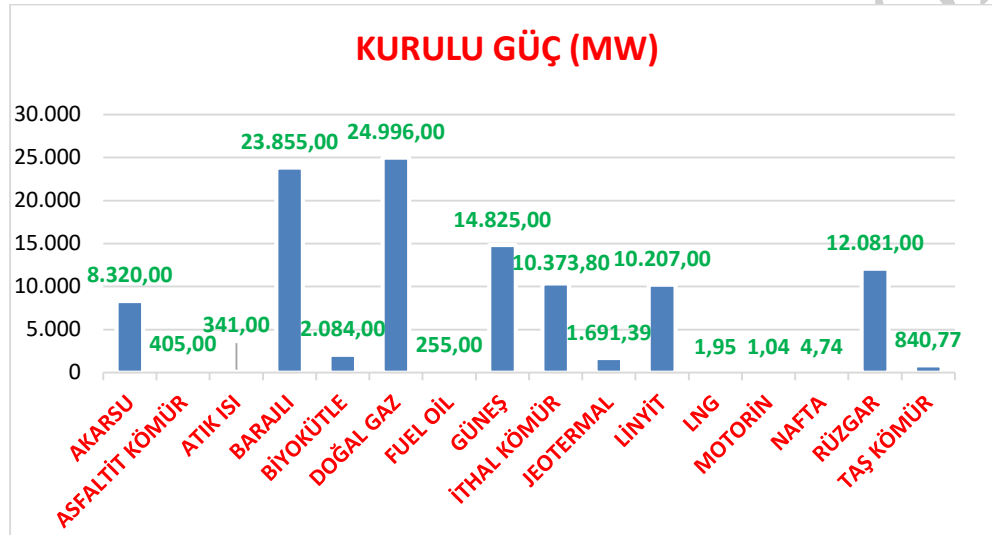
Şekil 1-Türkiye’de elektrik kurulu gücünün kaynaklara göre dağılımı –Mart 2024 Kaynak: TEİAŞ
