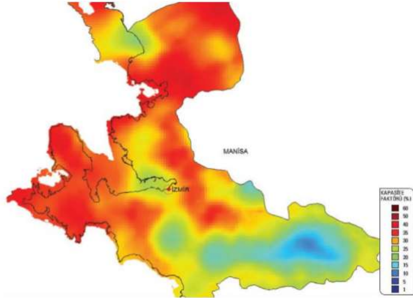
İzmir İli rüzgar enerjisi potansiyeli kapasite faktör haritası
