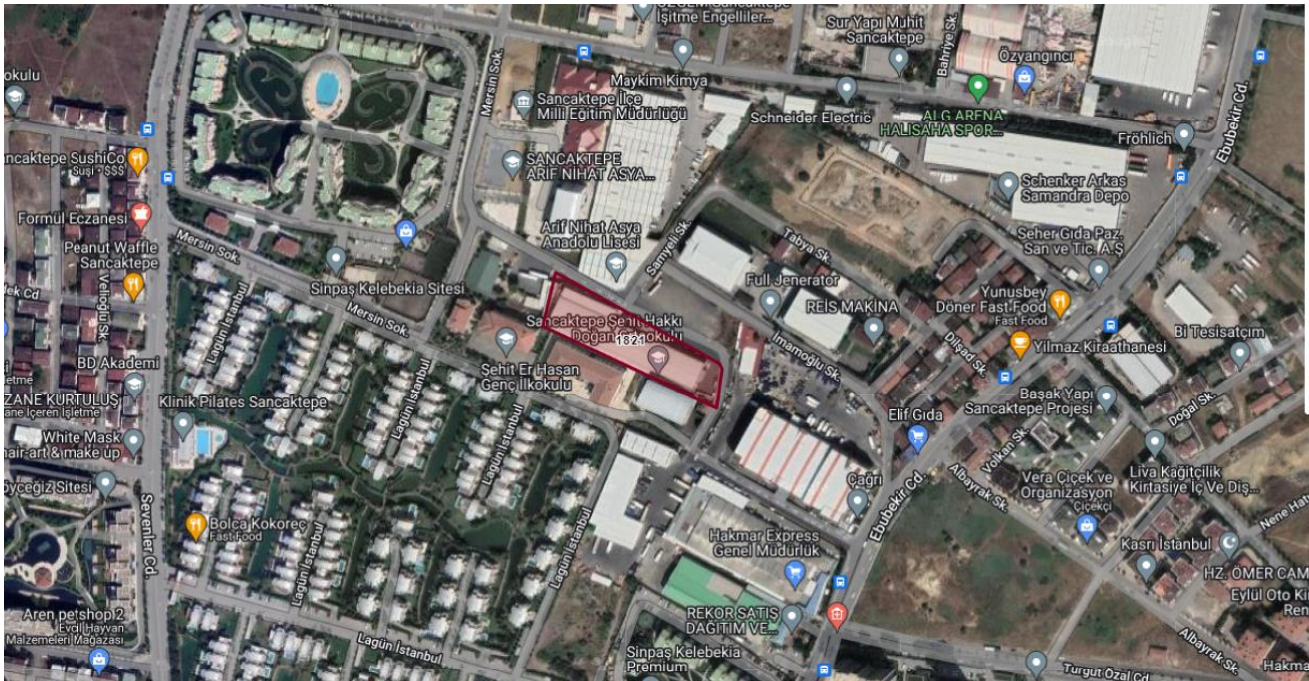
Uydu Görüntüleri
